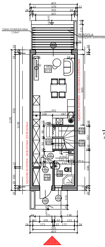
RZUT PARTERU- TYP A BM8
