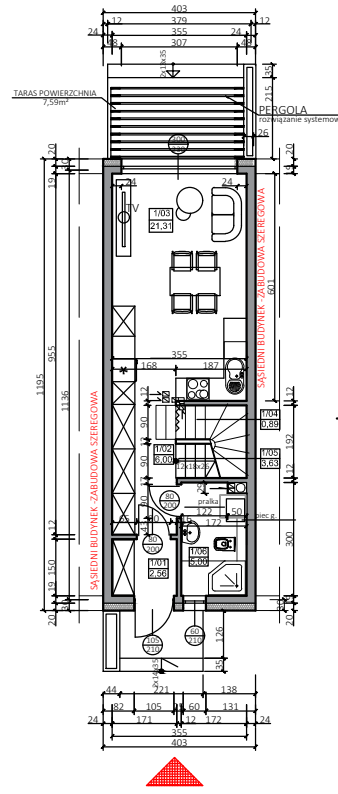
RZUT PARTERU- TYP A BM11
