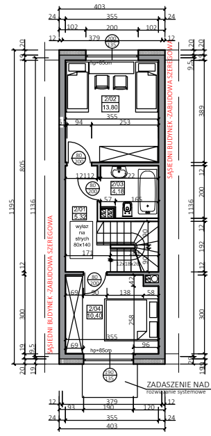
RZUT PODDASZA- TYP A BM11
